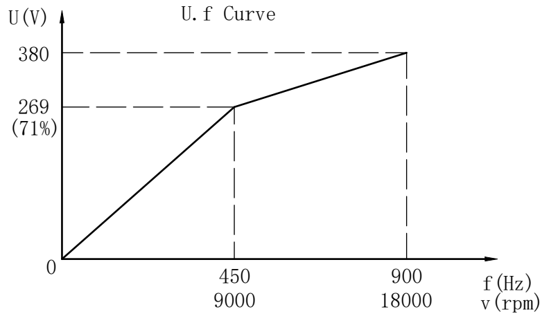
频压曲线
