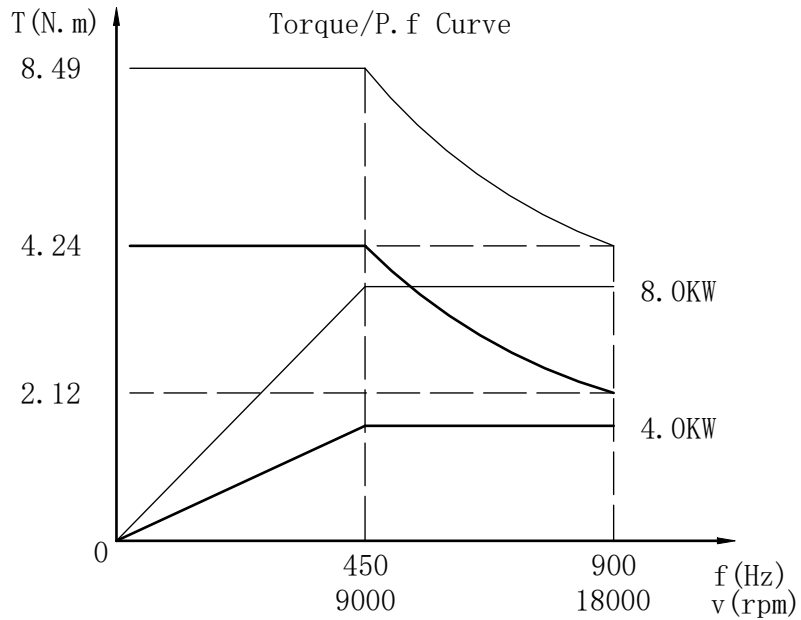
扭矩/功率曲线
